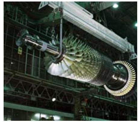
燃气轮机
